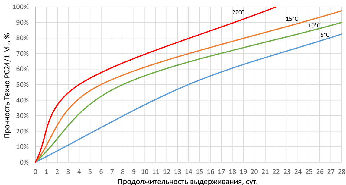
Рис.1. Прочность цементной штукатурки Техно РС24/1 ML в зависимости от температуры и продолжительности выдерживания.
